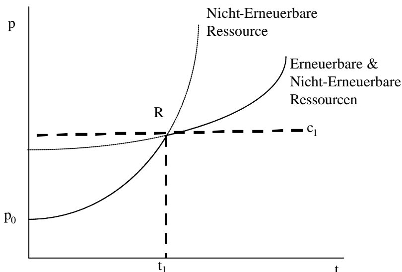
Abbildung 2-3 Betriebswirtschaftliche Kosten der Bereitstellung von Energie auf der Basis unterschiedlicher Energieträger
